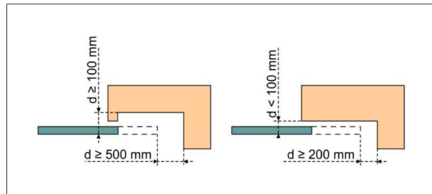
Ábra 1: Biztonsági távolság
