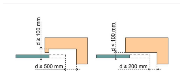
Illustratie 1: Veiligheidsafstand
